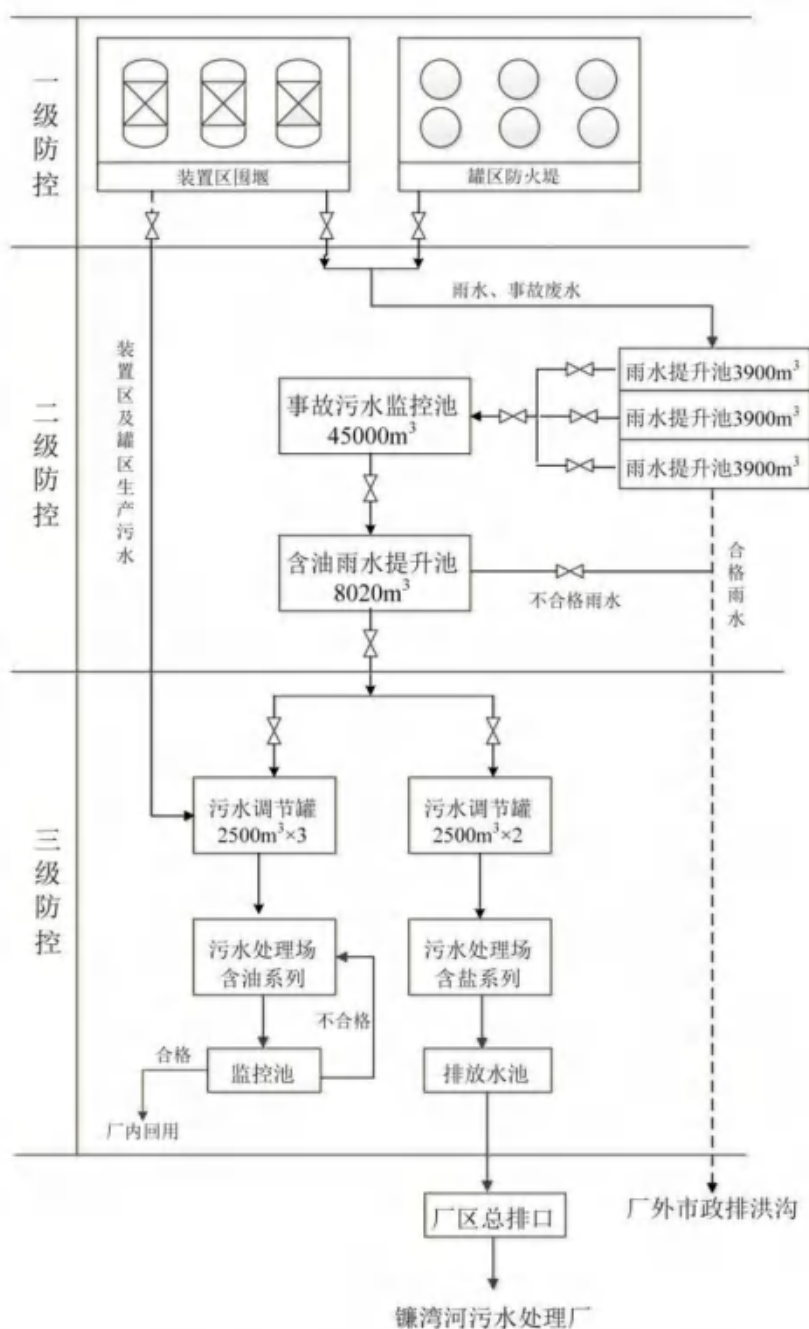
图 6.1-2 厂区事故废水三级防控系统示意图
