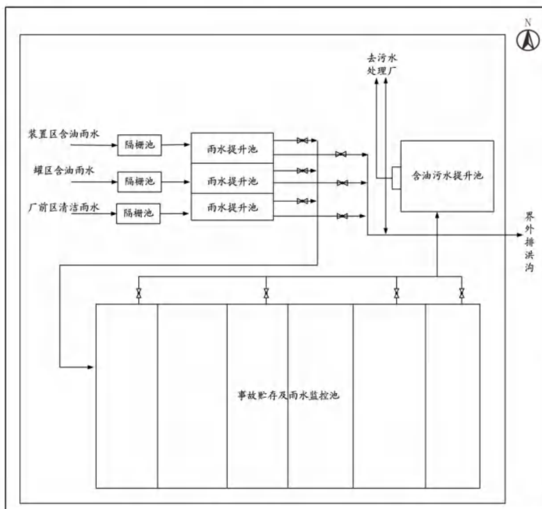
图 6.1-1 青岛炼化公司雨水处理系统示意图
