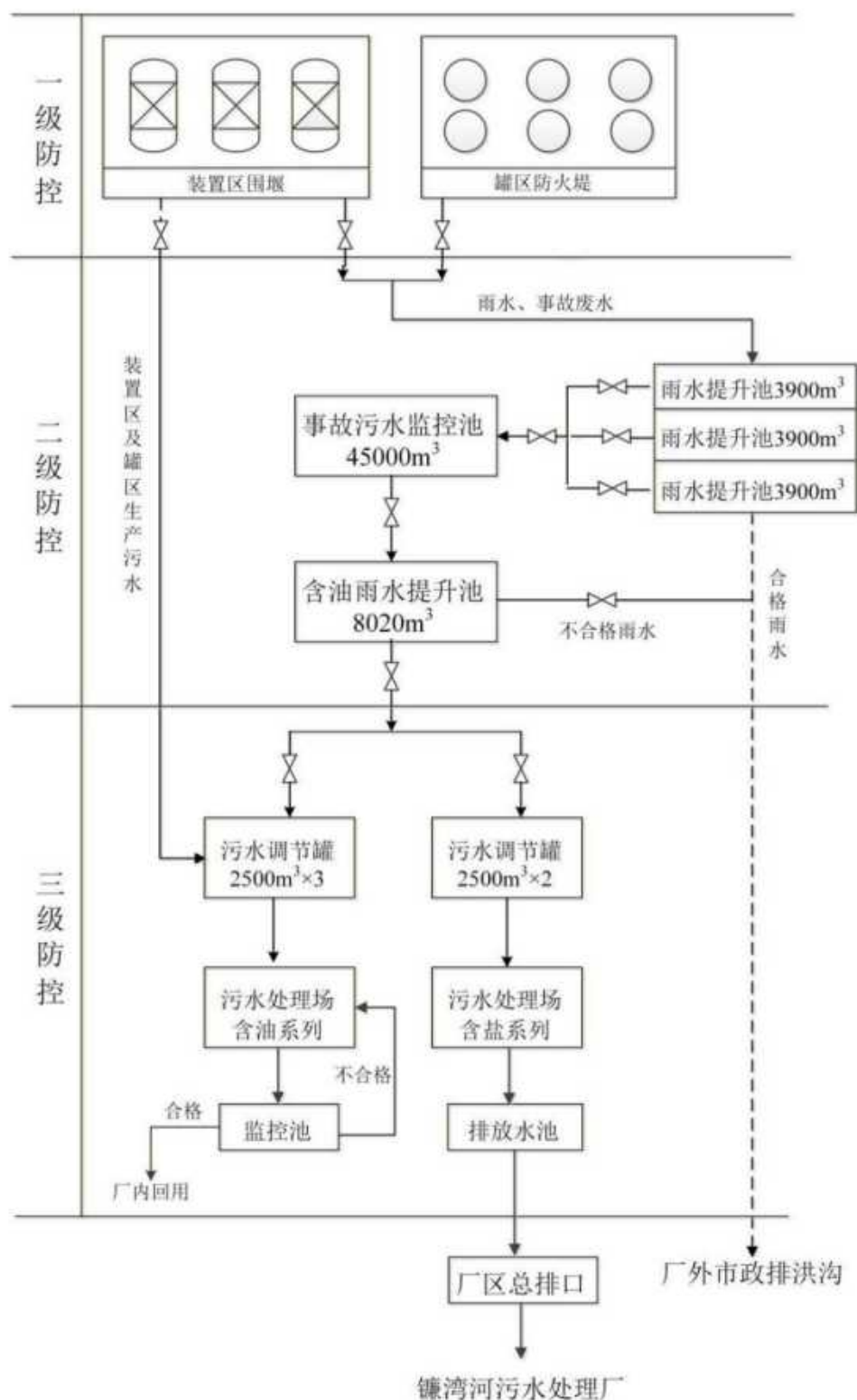
图 6.7-2 本项目事故废水三级防控体系示意图
