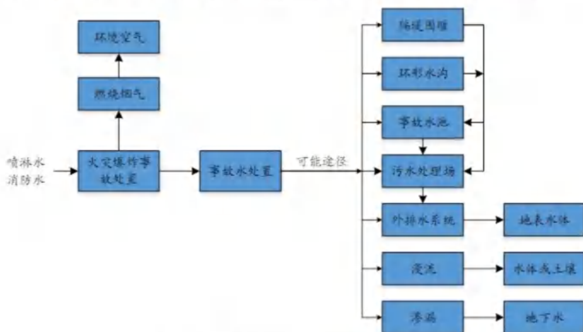
图 6.4-1 危险物质向环境转移的途径示意图
