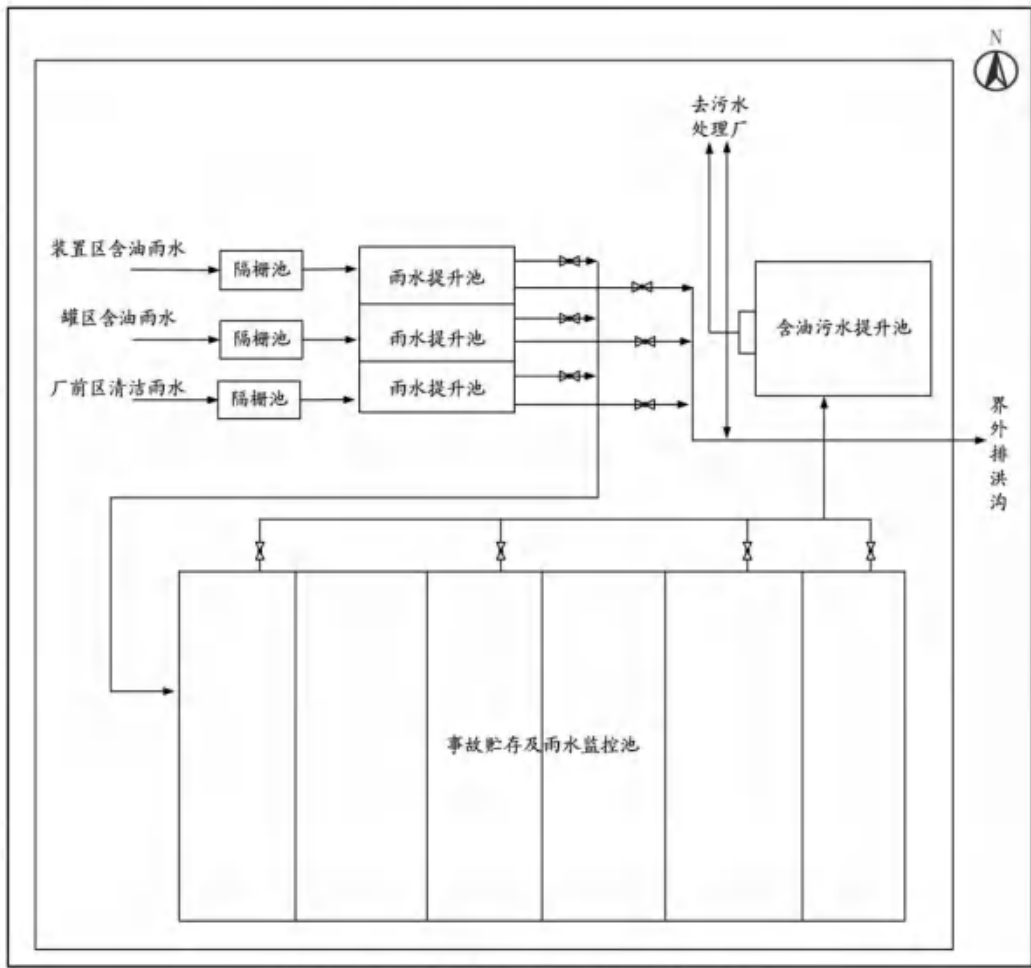
图 2.5-18 青岛炼化雨水处理系统示意图
