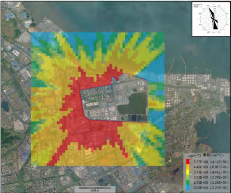
图 5.2- 29 新增 NMHC 小时平均贡献质量浓度分布图
