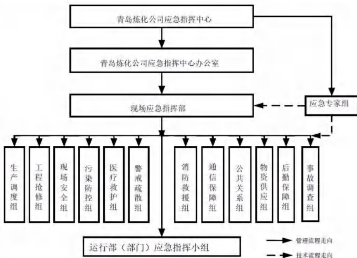
图 6.1-4 环境风险与应急管理组织机构图
