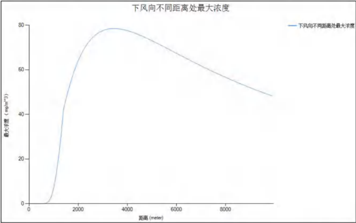
图 6.6-1 柴油储罐火灾事故下风向不同距离处次生 CO 最大浓度分布图（最不利气象）
