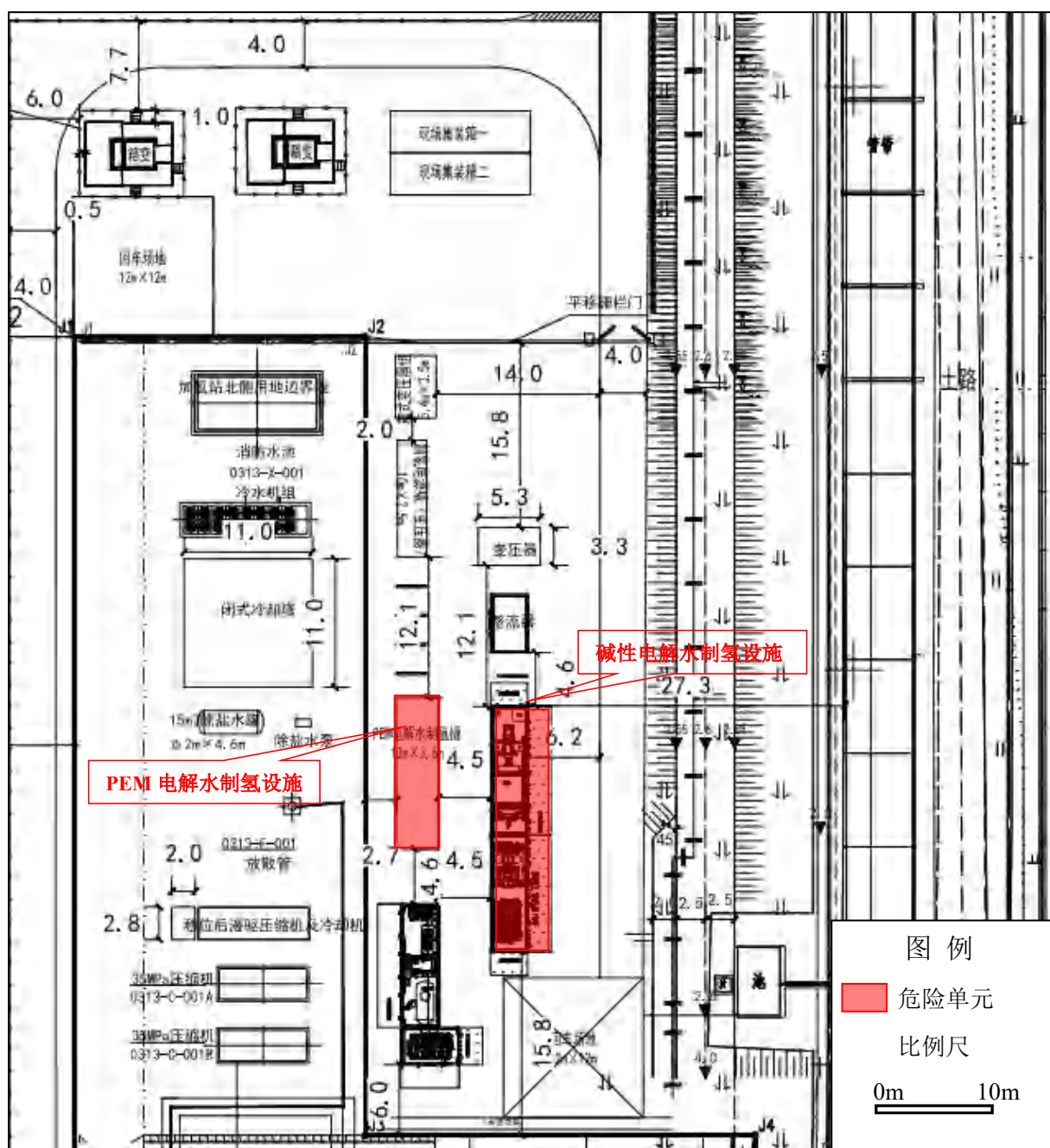
图 7.2-1 本项目危险单元分布图
