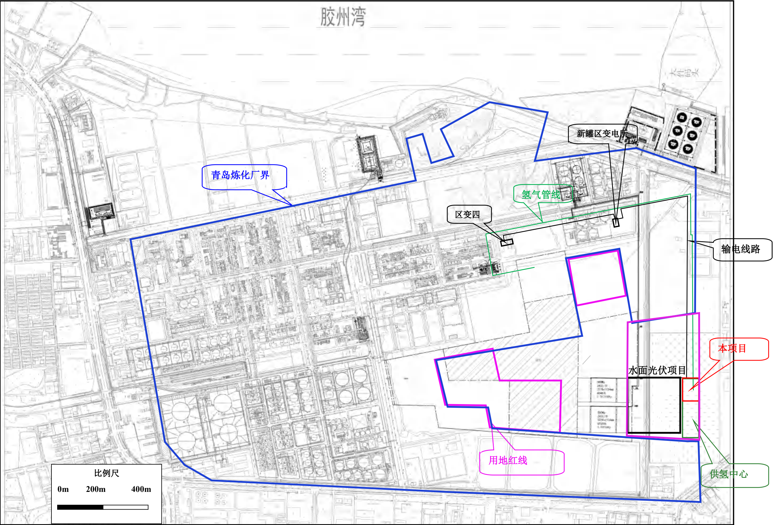
图 3.3-2 本项目工程位置图
