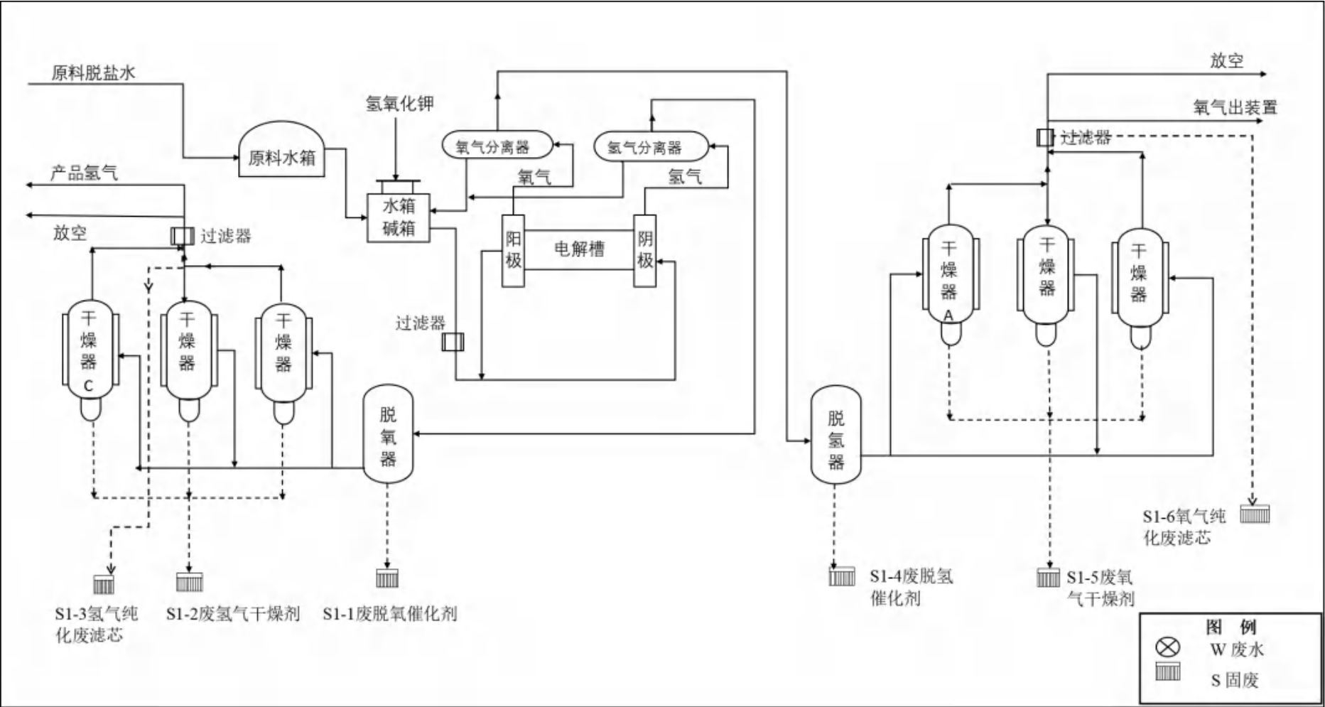
图 4.2-2 本项目工艺流程及产排污环节图
